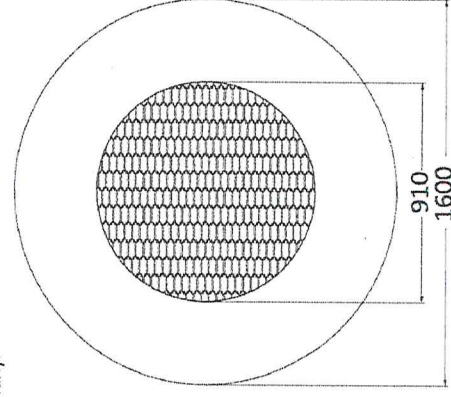
Рисунок 2. Габариты прыжкового устройства
