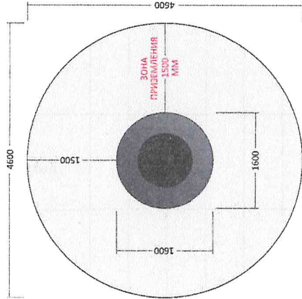
Рисунок 3. Зона приземления прыжкового устройства
