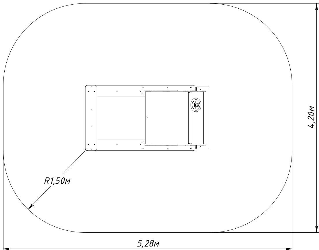
Рисунок 1 — Основные габаритные размеры
