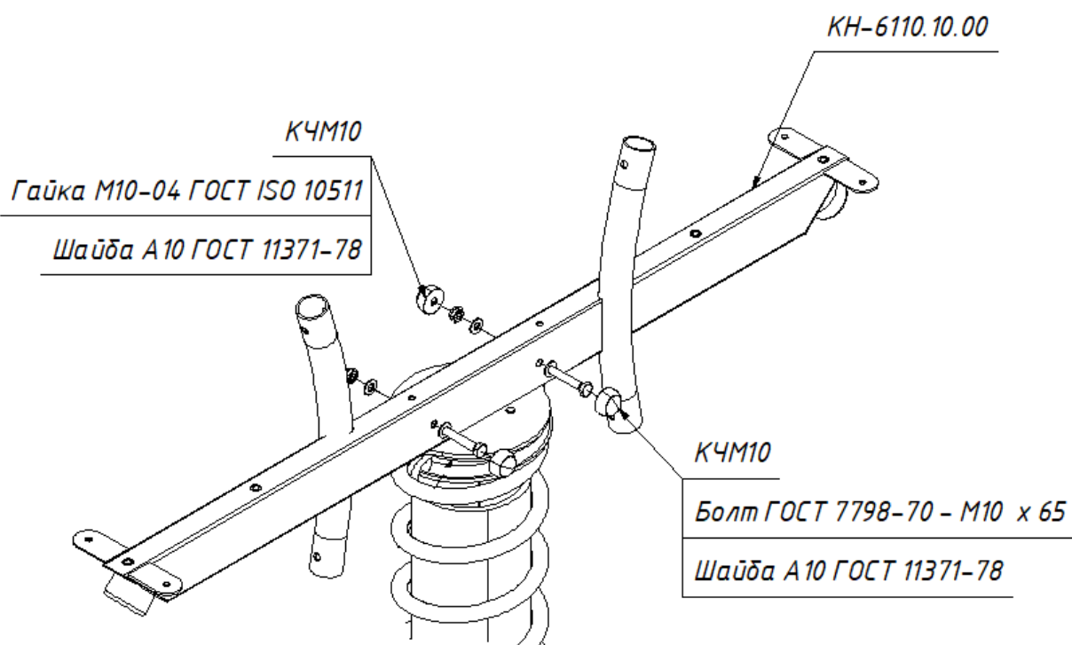
Рис. 12 Соединение балки и основания
