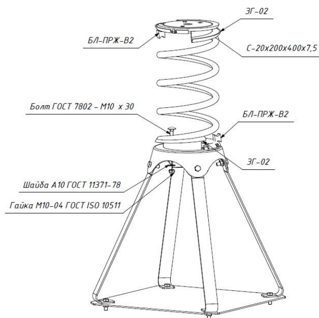
Рис. 9 Схема установки пружины
