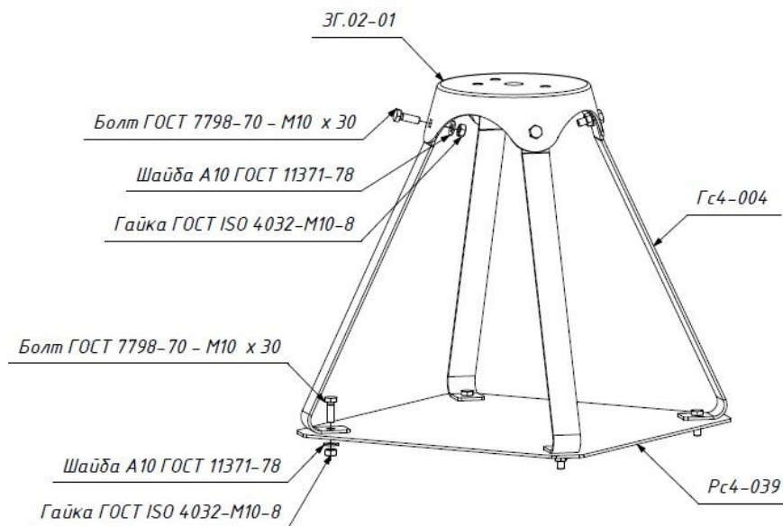
Рис. 7 Схема сборки закладной качалки
