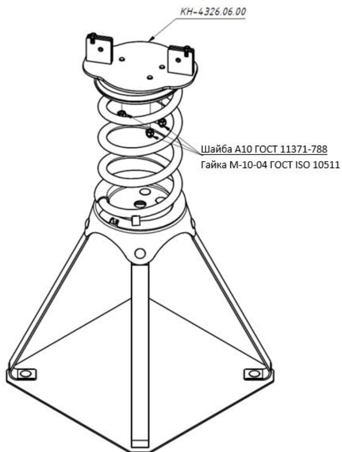
Рис. 11 Соединение балки и основания
