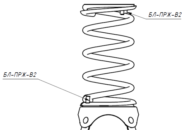
Рис. 8 Схема установки вставок БЛ-ПРЖ-В2
