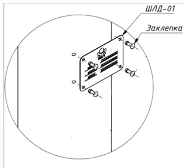
Рис. 16 Схема установки шильдика
