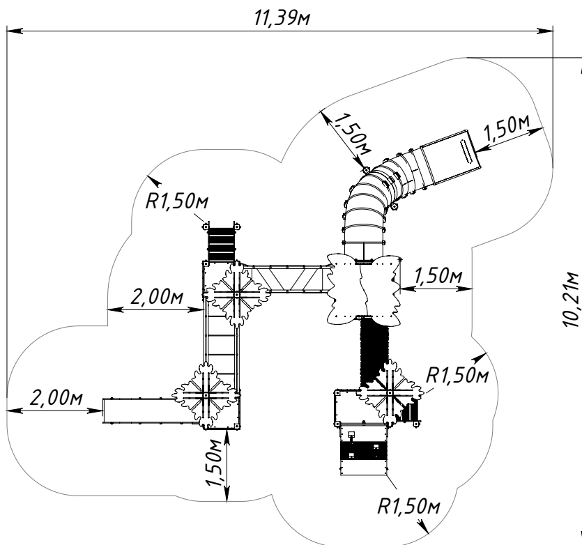
Рисунок 1 — Основные габаритные размеры
